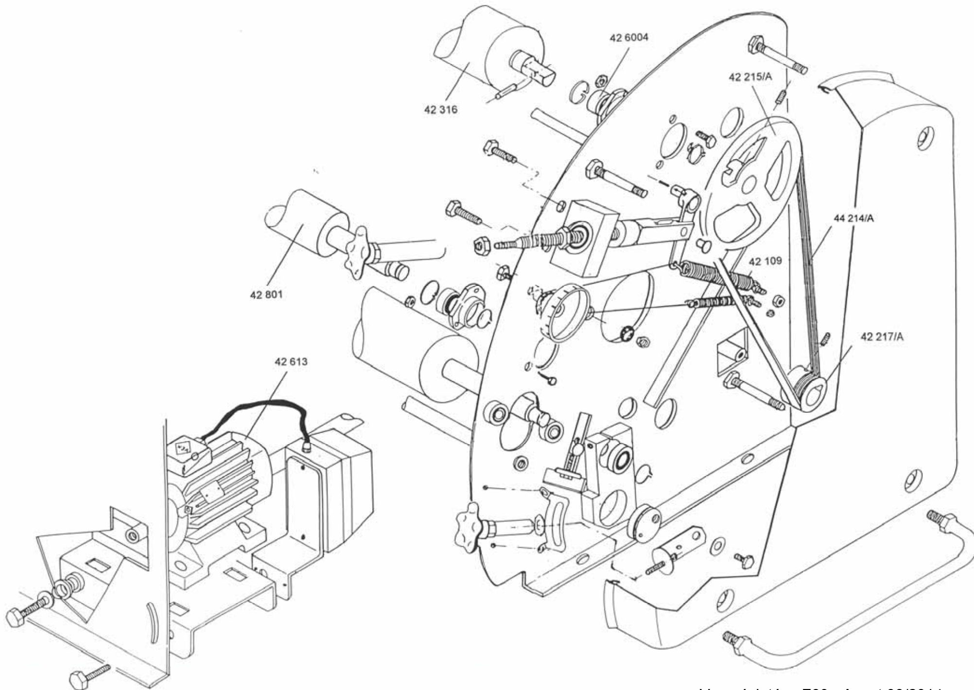
Vues éclatées F60 - Avant 09/2014
